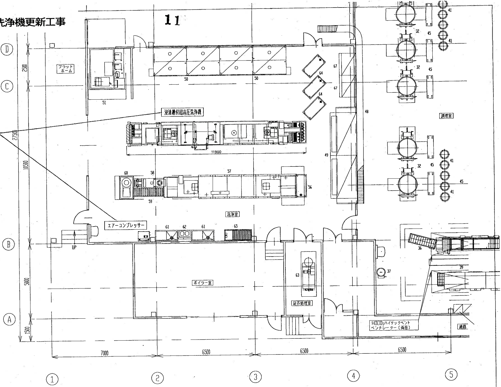
厨房設備器具配置図
