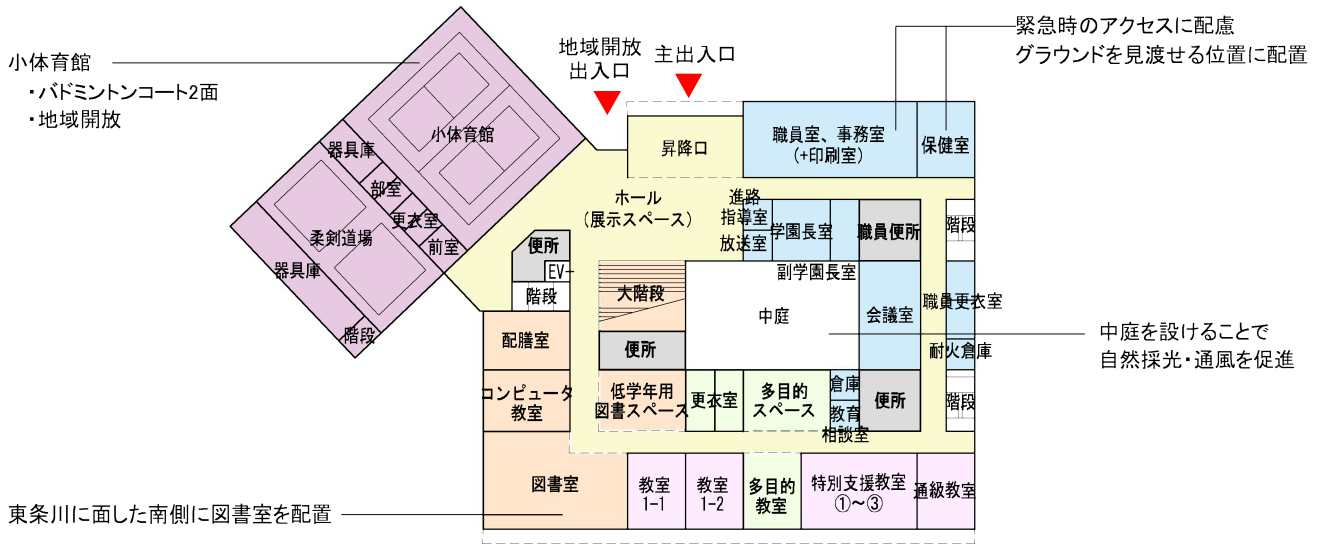
1階平面図
