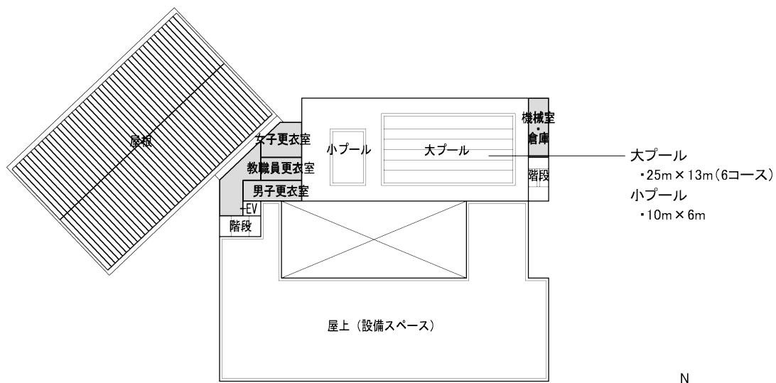
4階平面図
