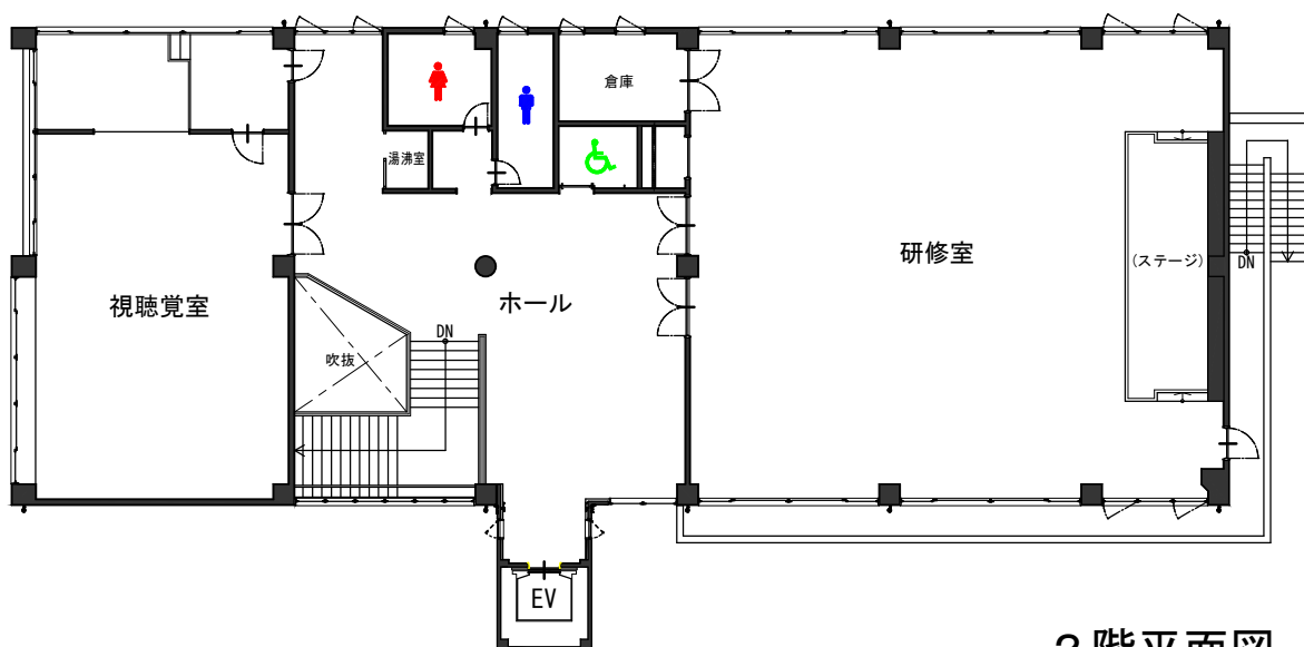
2階平面図
