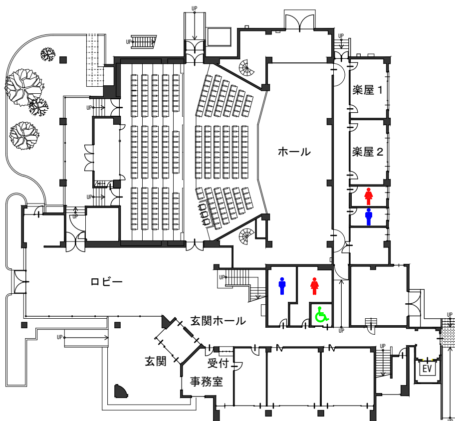
1 階平面図
