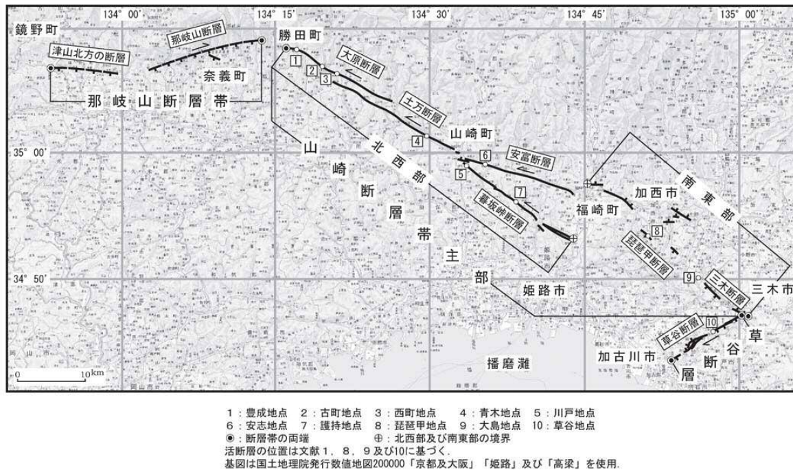
図 山崎断層帯の活断層位置図
