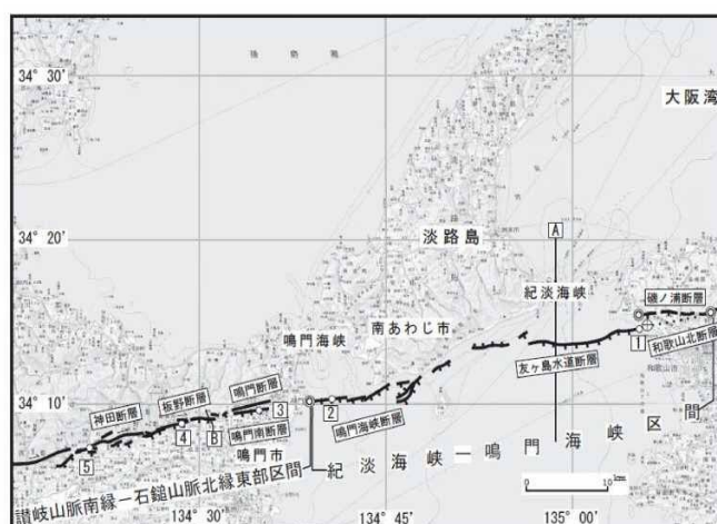
図2-2 中央構造線断層帯の活断層位置と主な調査地点 1：紀淡海峡地点 2：鳴門海峡地点 3：段岡・大代地点 4：川端A、B地点 5：熊谷寺東南地点 A：文献39 B：文献34 活断層の位置は文献4、11、14、17、22に基づく。 .....：活断層が地表に現れていない区間 ◎：活動区間の両端および境界 ⑤：紀淡海峡-鳴門海峡の活動区間のうち、第四紀後期における活動性が確かめられている区間の東端 基図は国土地理院発行数値地図200000「和歌山」及び「徳島」を使用。
