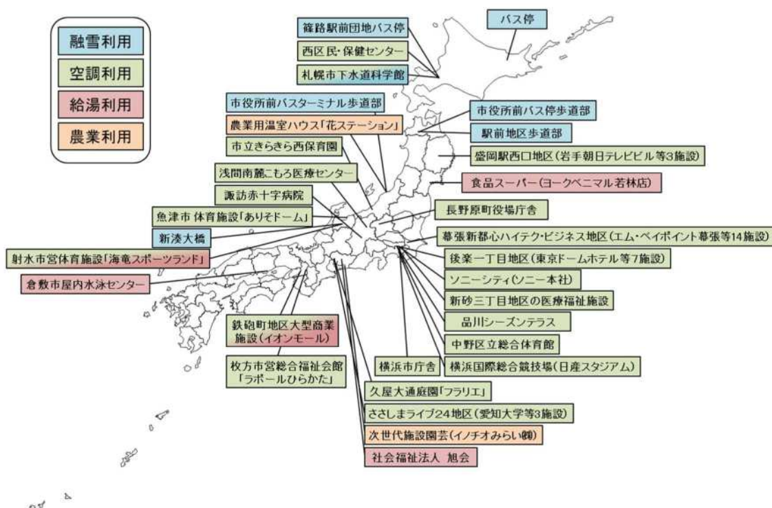
図2-11 国内における下水熱利用の事例(令和2年8月末時点)
