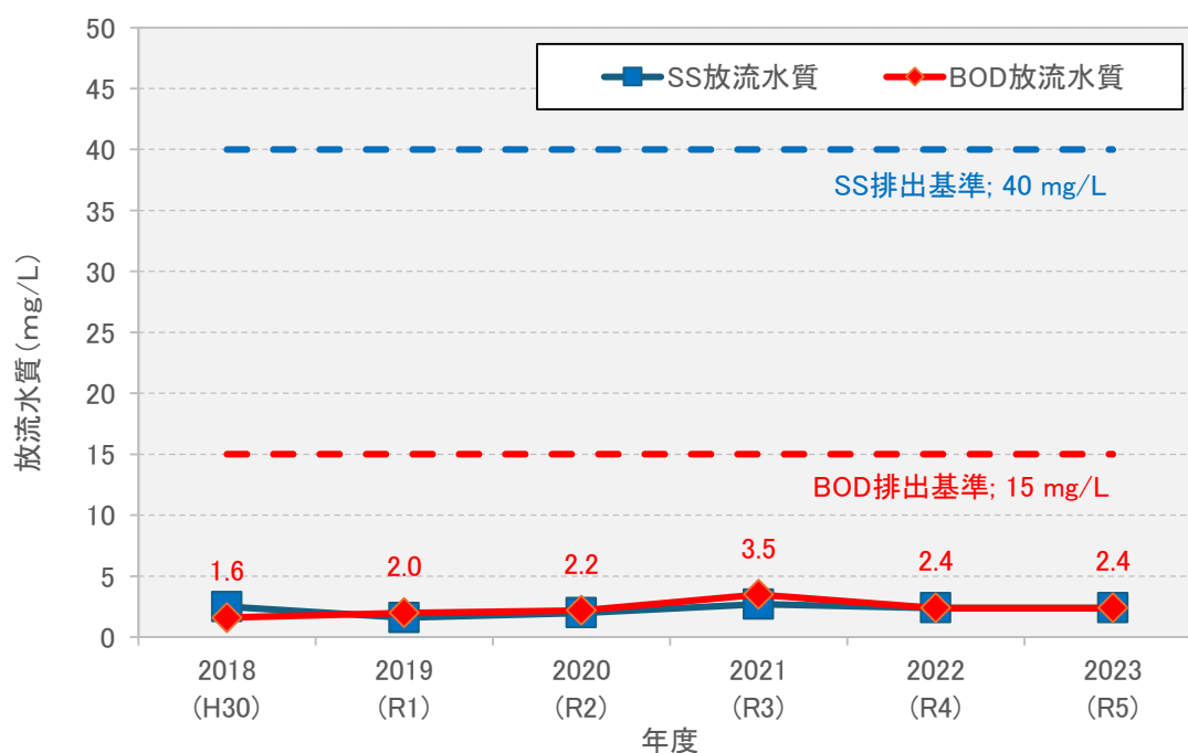
図2-2 せせらぎ東条の放流水質推移
