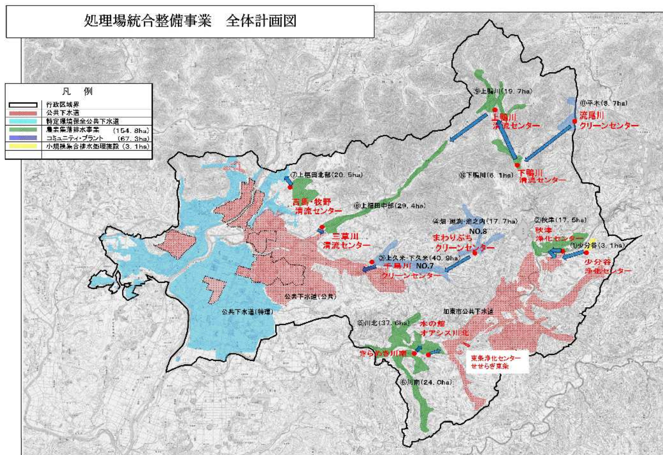
図2-8 処理場施設統合 全体計画図
