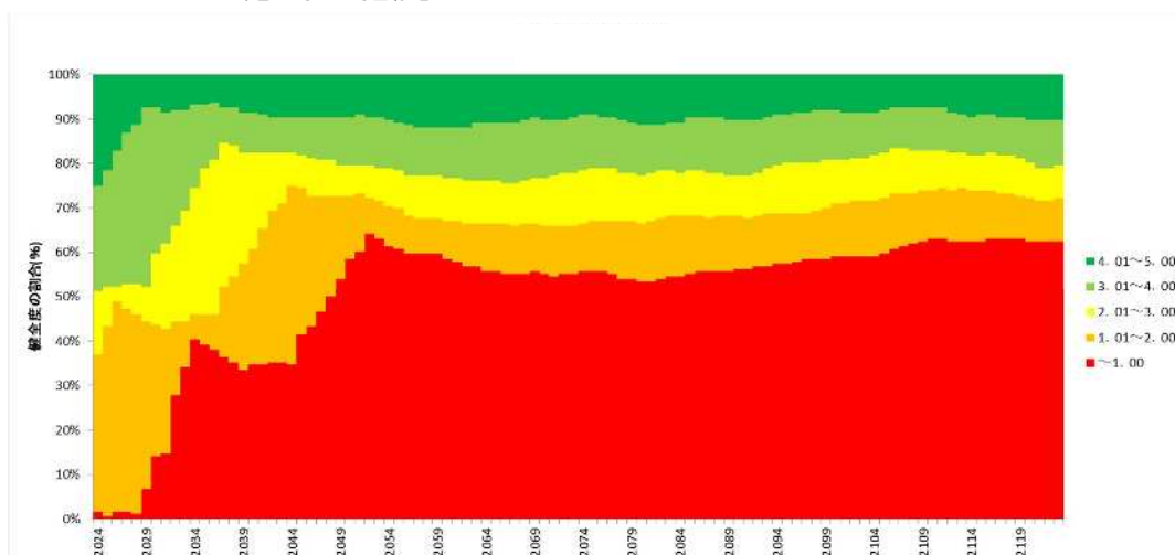
図3-14 マンホールポンプの事業費、リスク点数、健全度の推移 （シナリオ7：予算制約シナリオ4（年間事業費400万円 ※実現可能な予算によるシナリオ））
