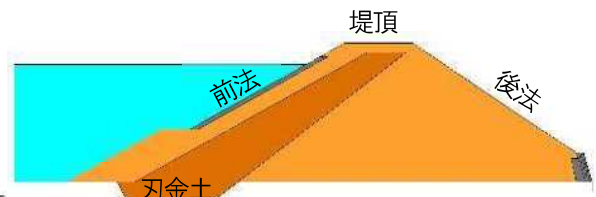
図3:ため池の断面図(傾斜コア型)
