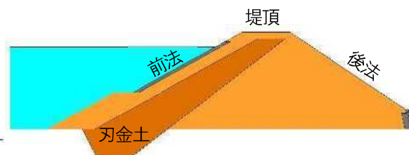
図3：ため池の断面図(傾斜コア型)
