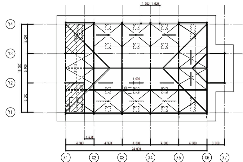
天井伏図 (改修前) 1/200
