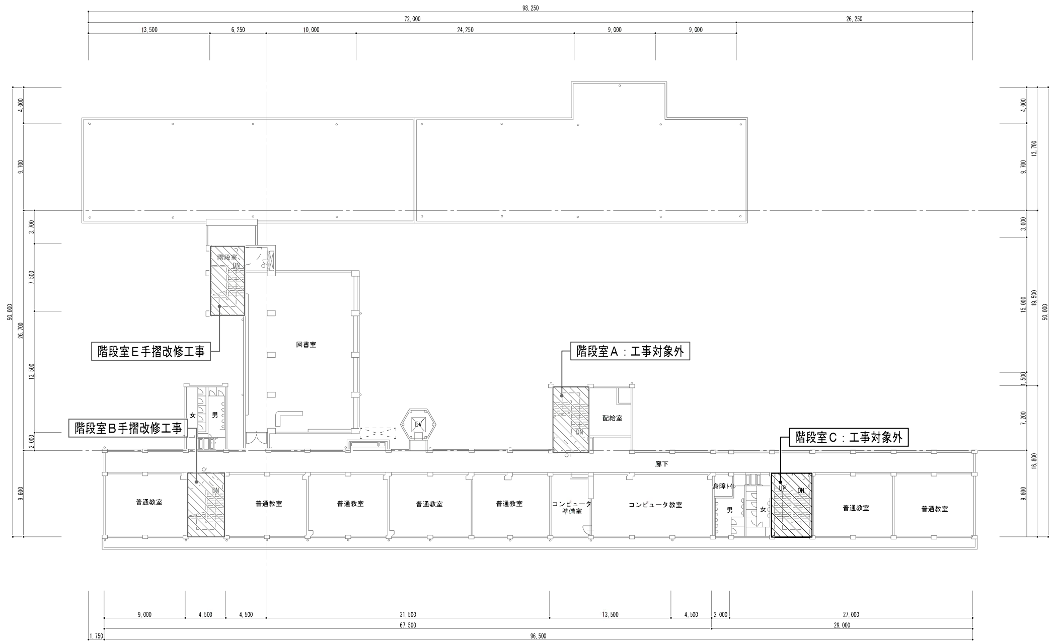
3階平面図 (S=1/300)
