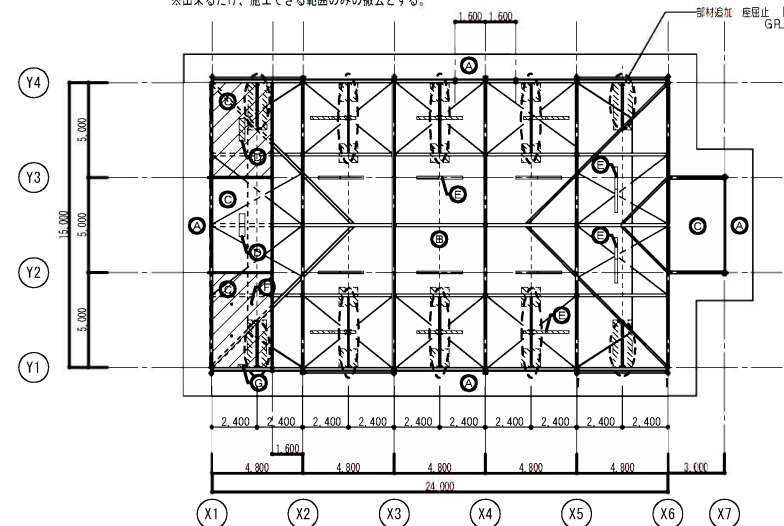
天井伏図 (改修後) 1/200
