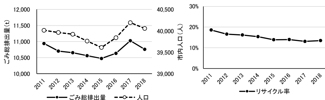
図 本市のごみ総排出量と人口の推移（左）、リサイクル率の推移（右）
