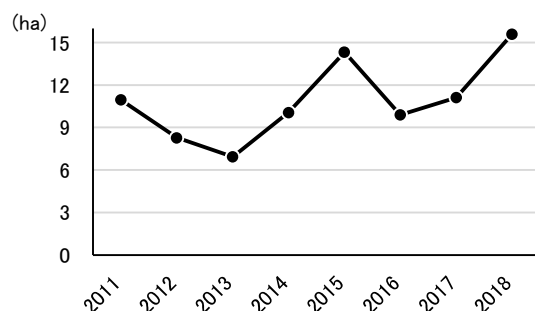
図 市内の遊休農地面積の推移
