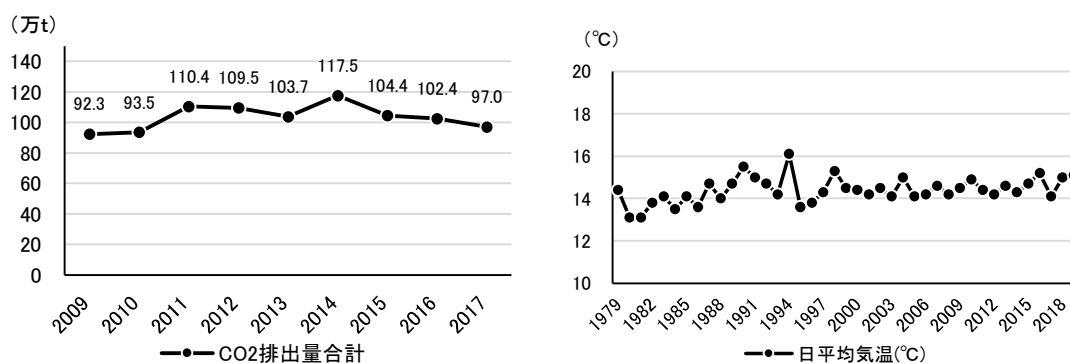
図 市内の二酸化炭素排出量の推移（左）、西脇地点の日平均気温の推移（右） （環境省、気象庁）
