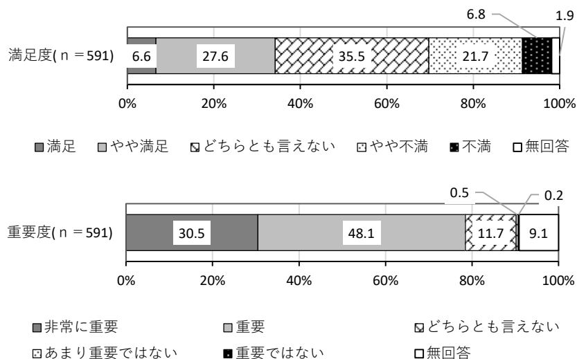
図 市民アンケート結果（川や水路、ため池のきれいさに対する満足度（上）と重要度（下））
