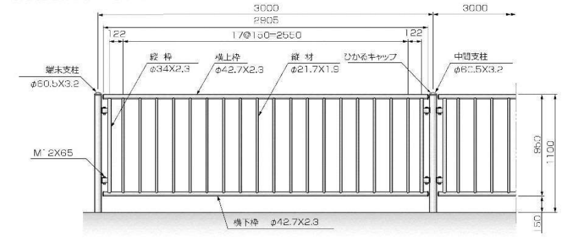
防護柵参考図
