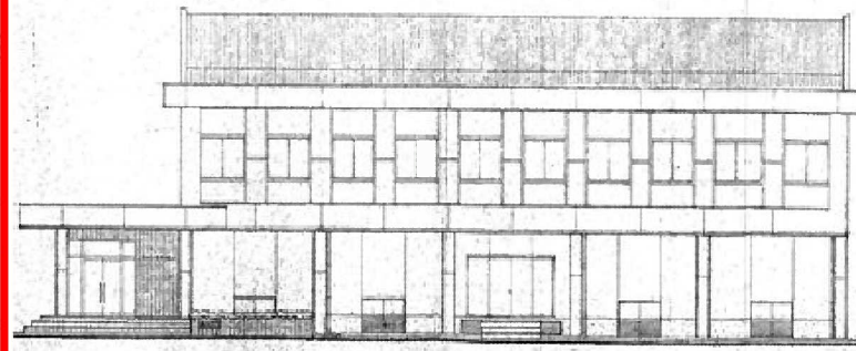
立面図（西側）
