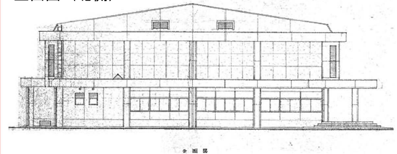
立面図（北側）
