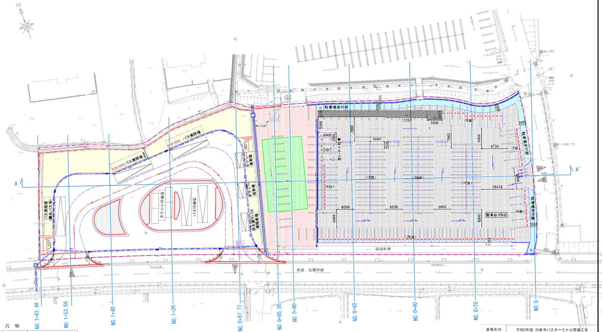
計画平面図
