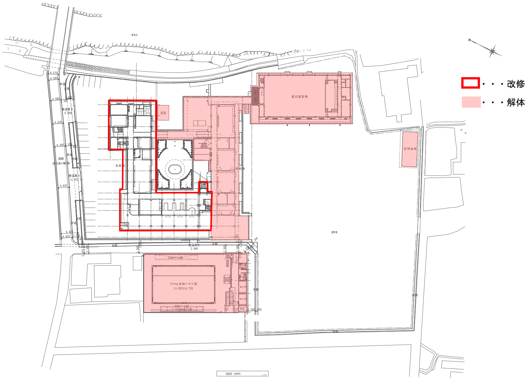
旧東条東小学校施設転用工事図面
