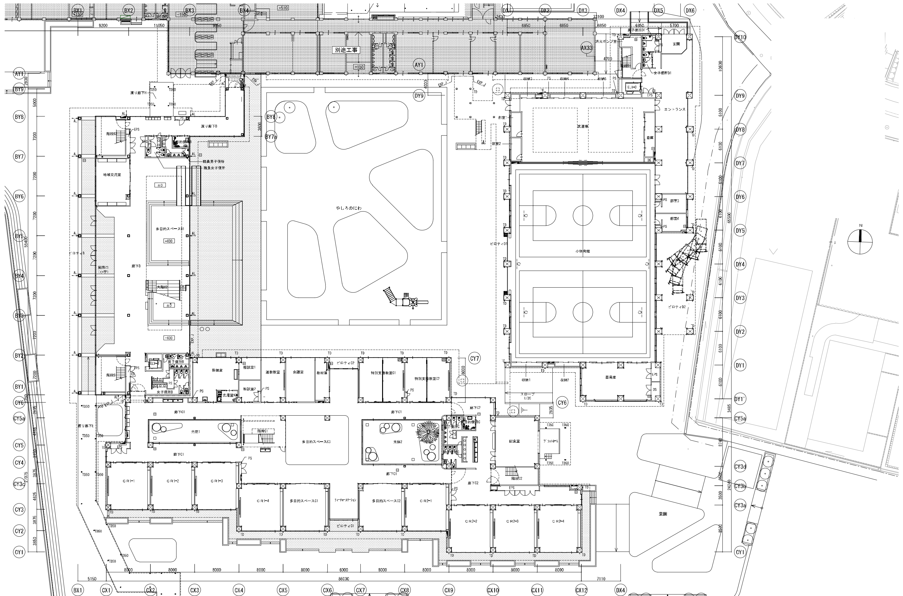
加東市社地域小中一貫校建設工事 1階平面図
