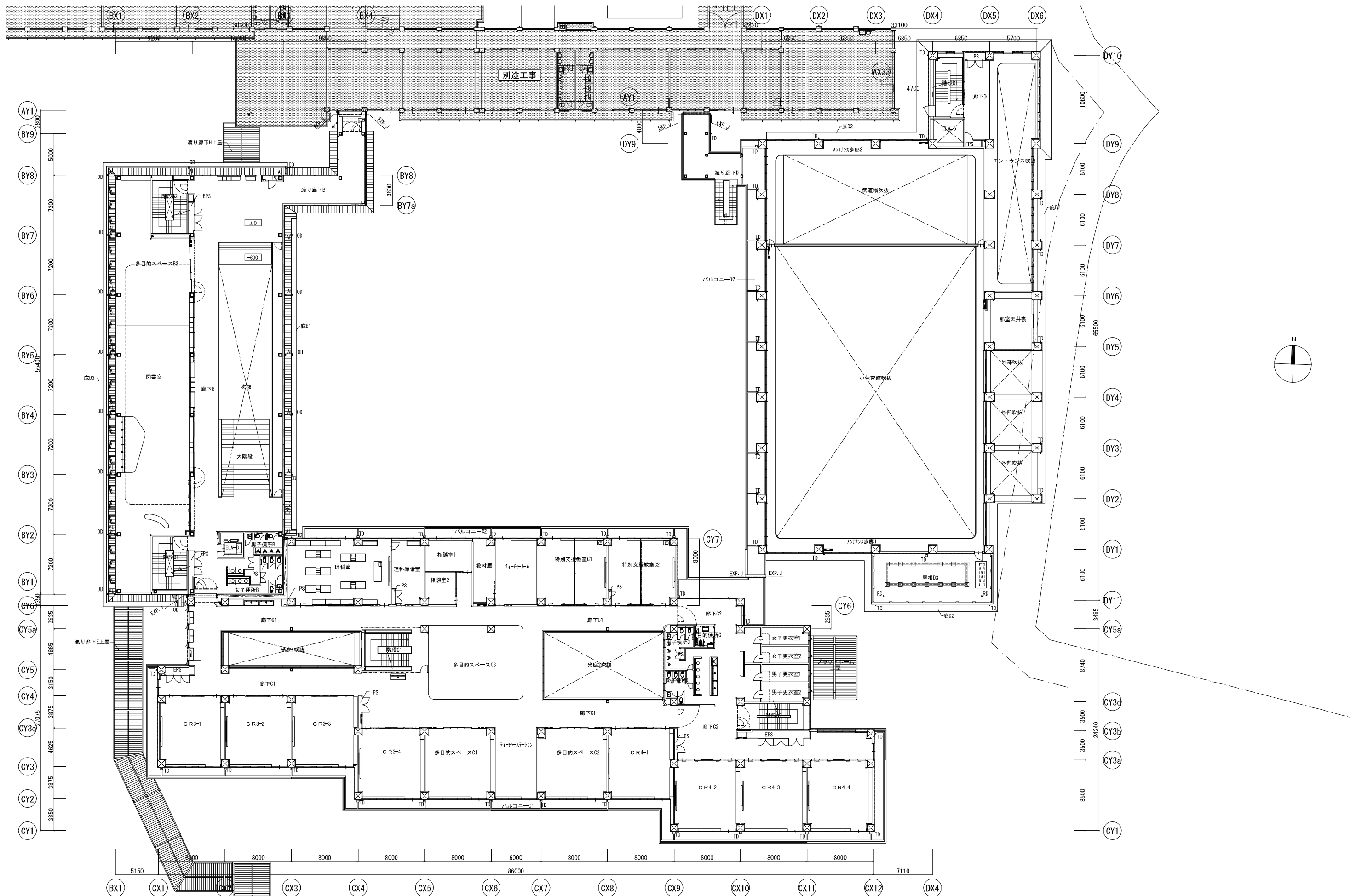
加東市社地域小中一貫校建設工事 2階平面図
