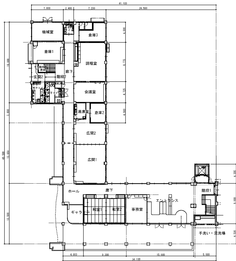
1階平面図
