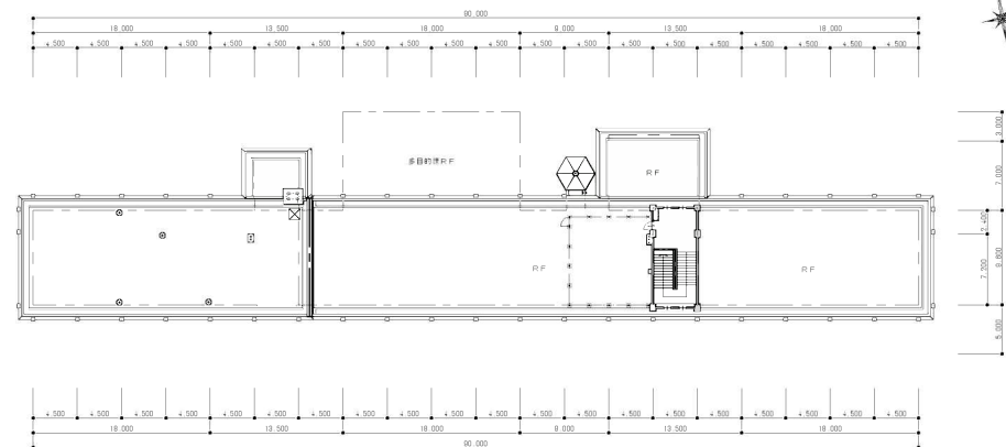
R階平面図 (S=1/600)
