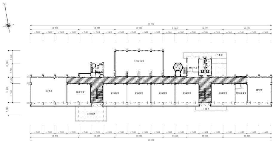
2階平面図 (S=1/600)
