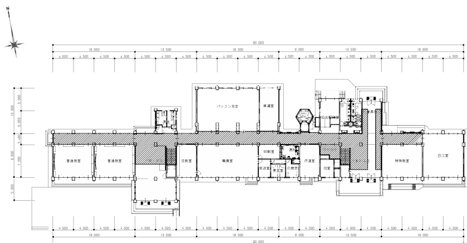
1階平面図 (S=1/600)
