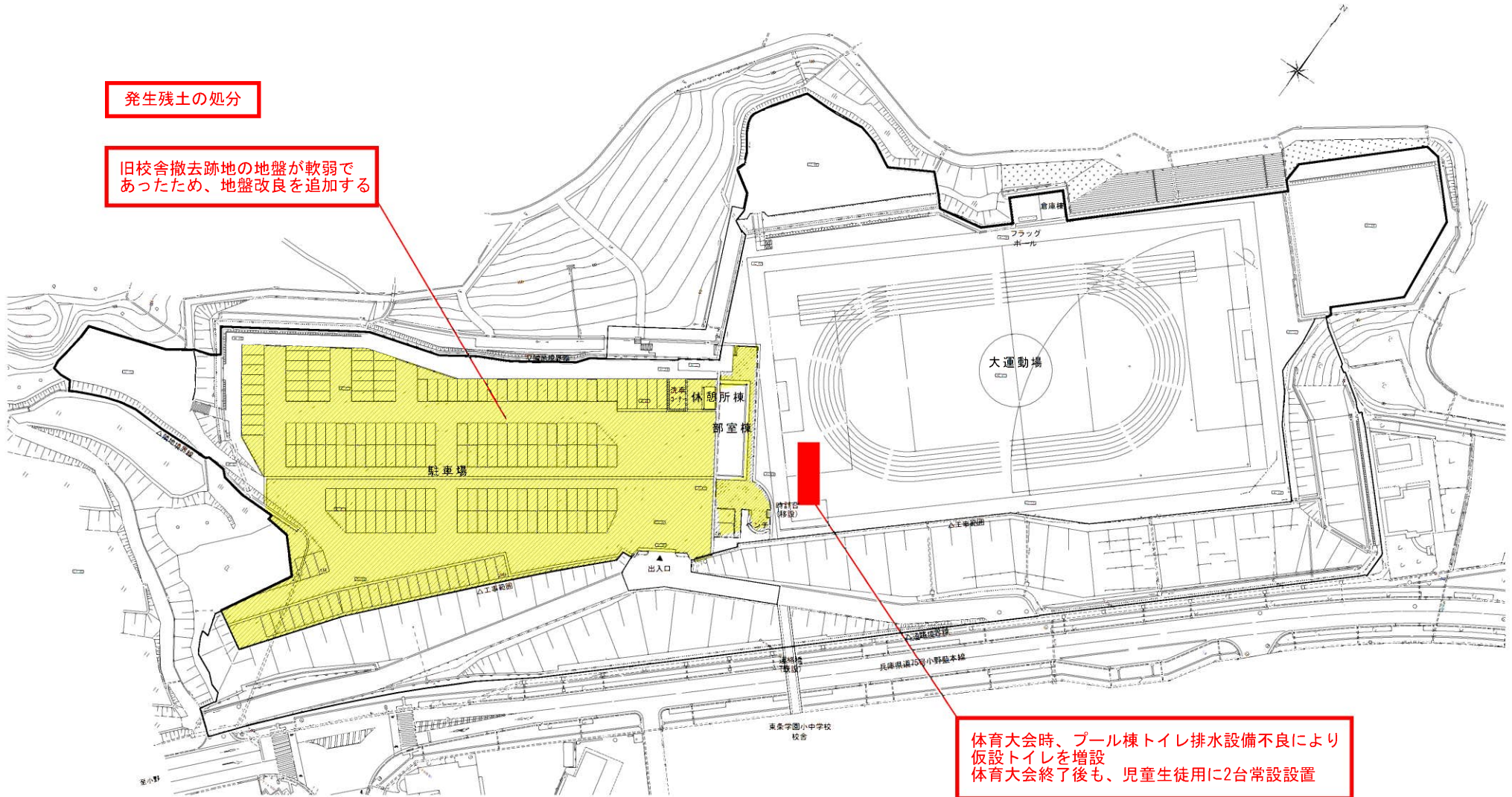
配置図 S=1/1000
