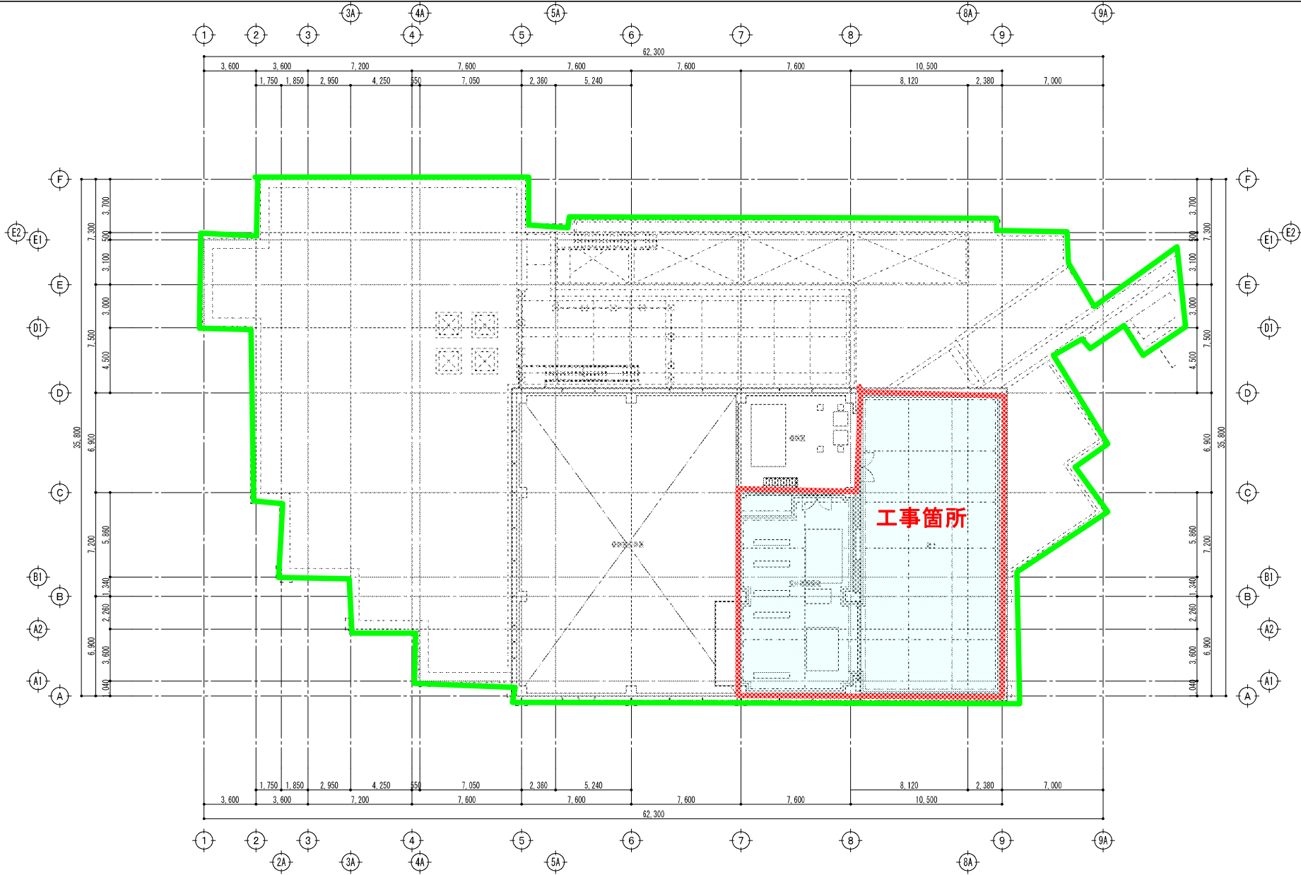
4階平面図 (S=1/250)
