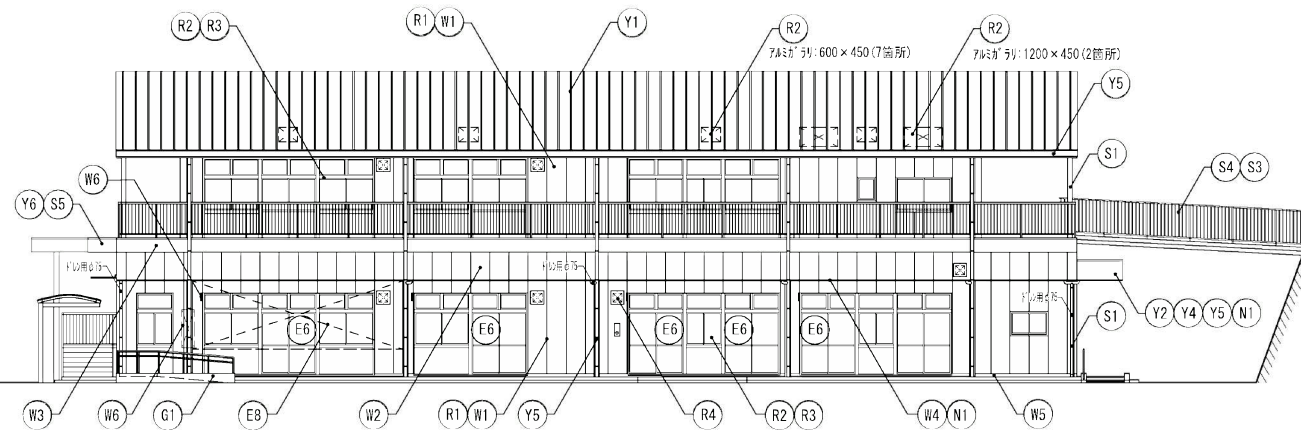
【改修後】西面 立面図 S=1:150
