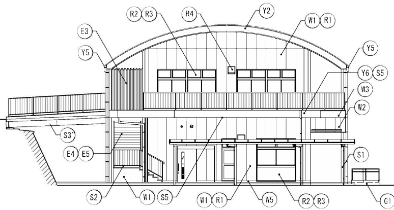
【改修後】北面 立面図 S=1:150
