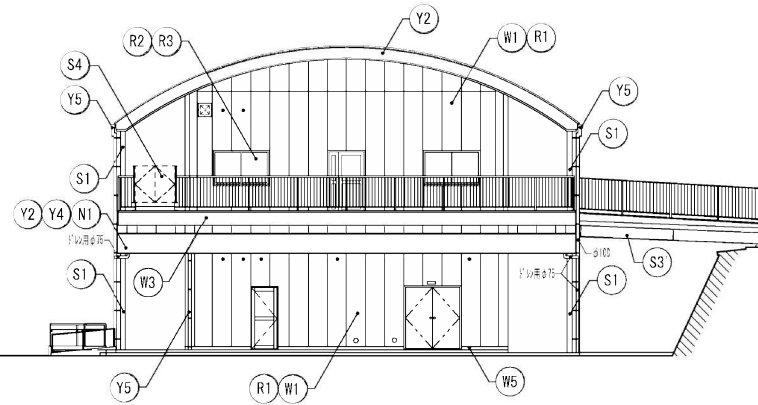
【改修後】南面 立面図 S=1:150
