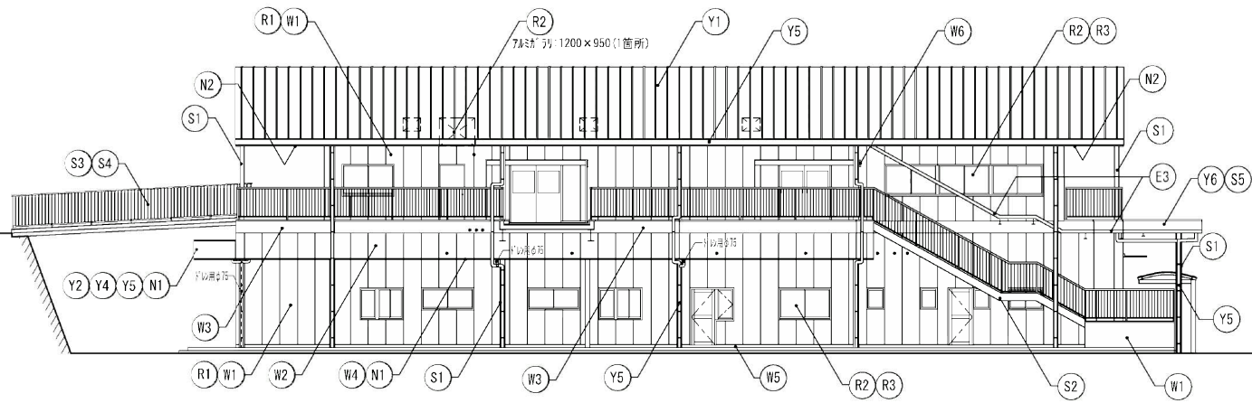
【改修後】東面 立面図 S=1:150
