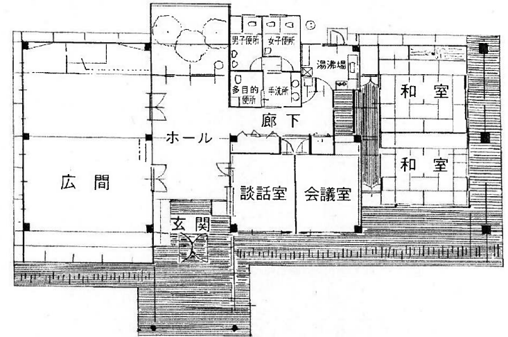
コミュニティセンター東条会館平面図
