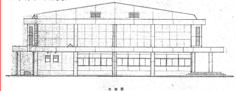
立面図（北側）
