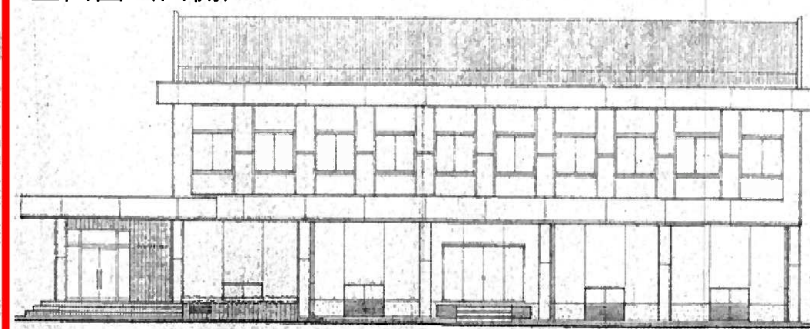
立面図（西側）
