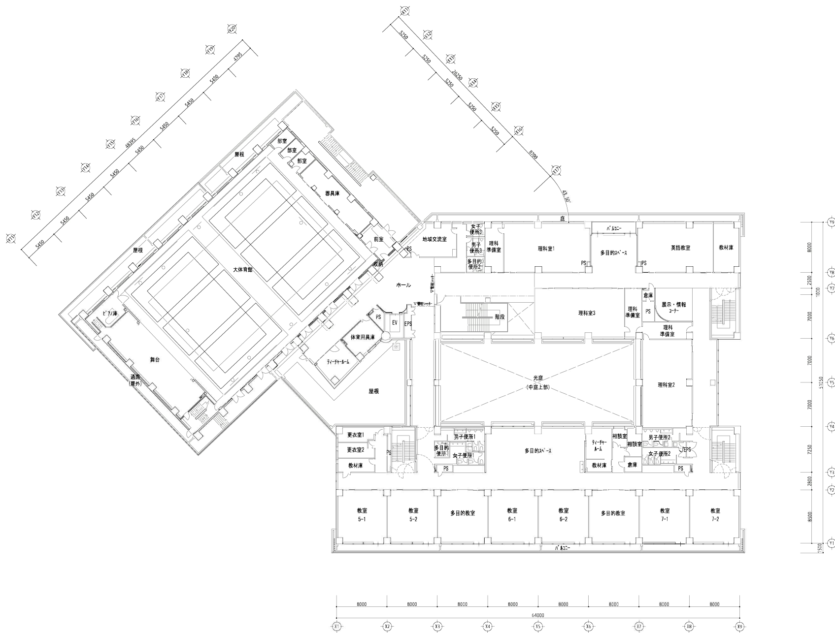
3階平面図
