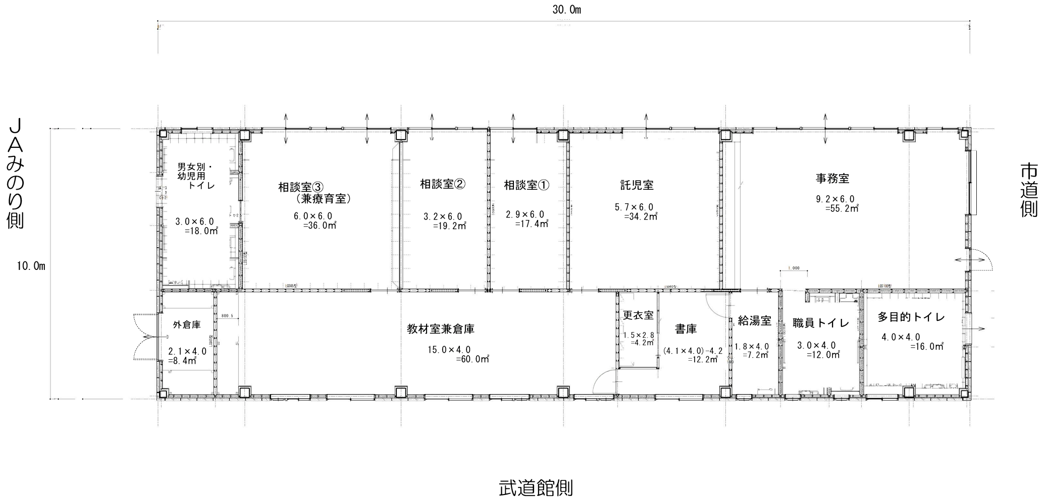
1 階平面詳細図
