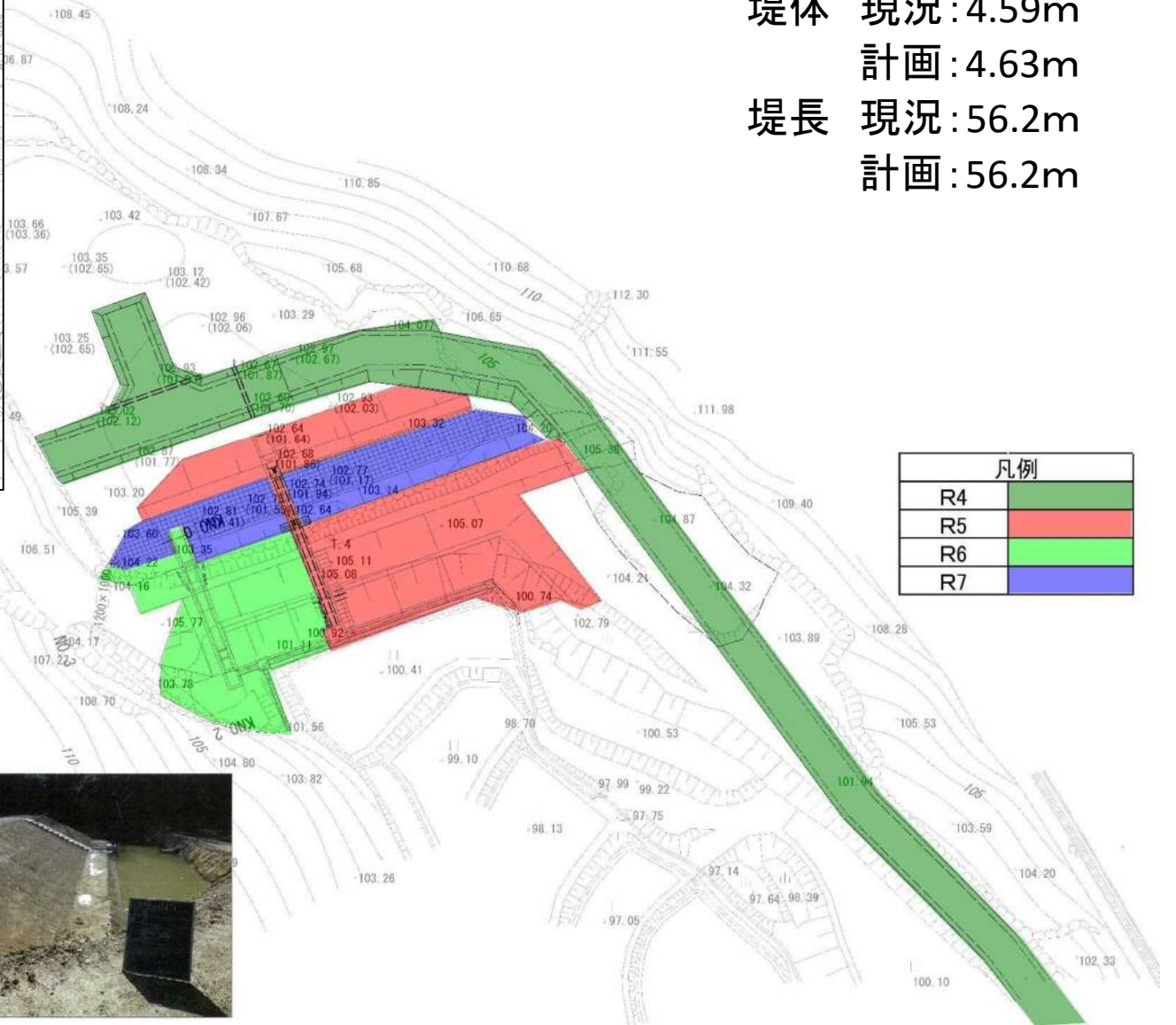
計画平面図
