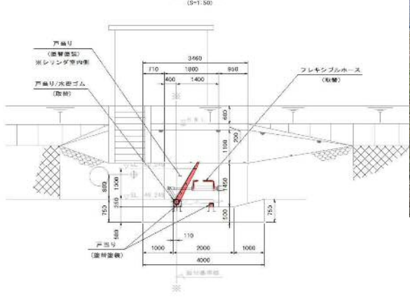
側断面図 (S=1/30)
