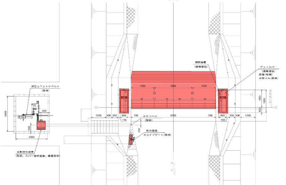
正面図 (S=1/30)
