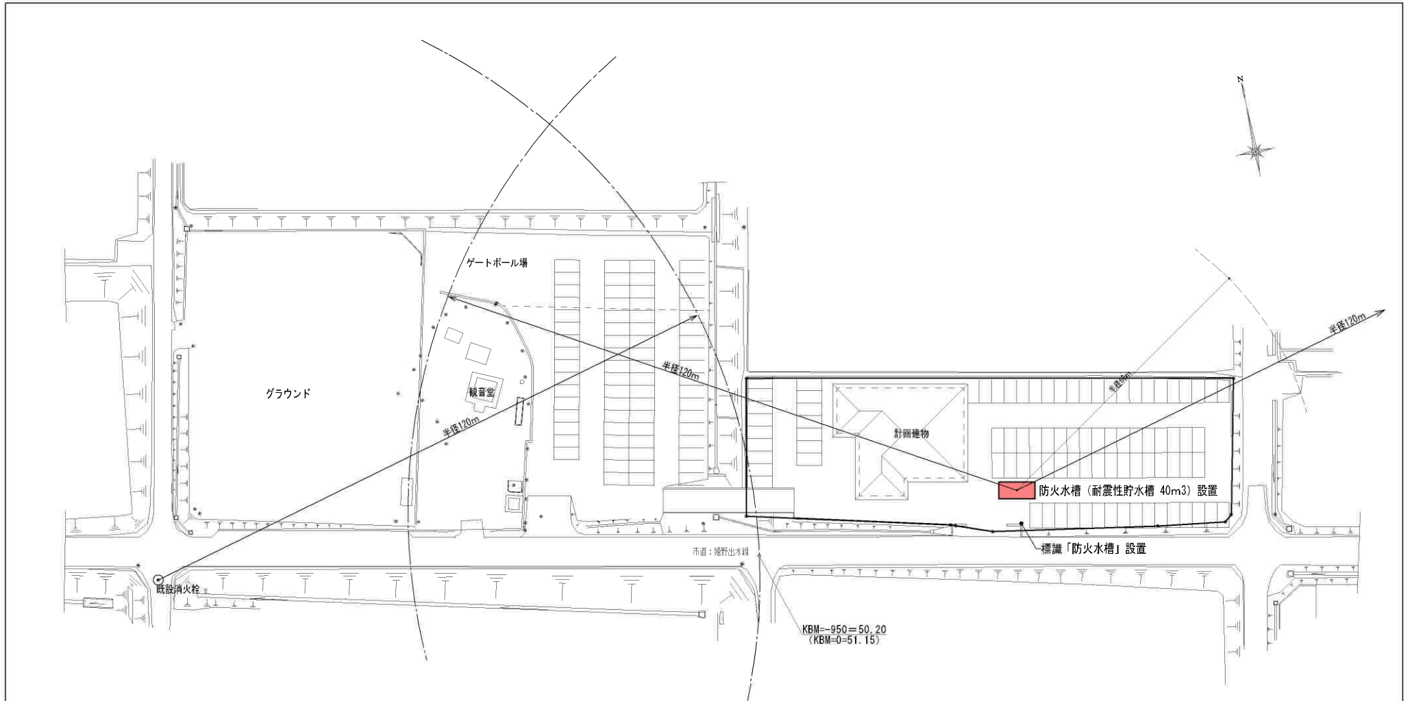
全体計画図 (S=1/700)
