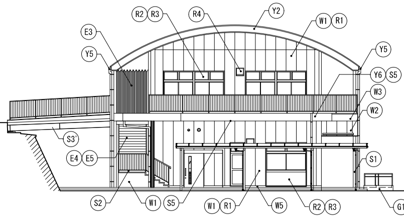
【改修後】北面 立面図 S=1:150
