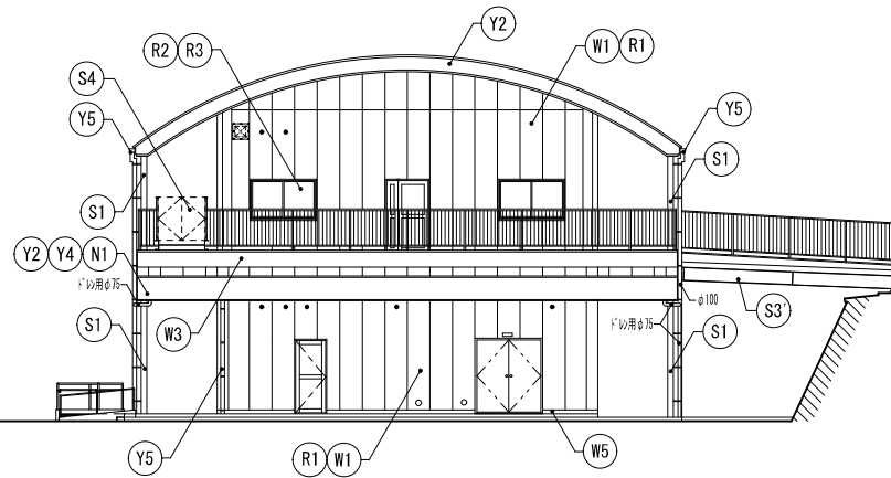
【改修後】南面 立面図 S=1:150
