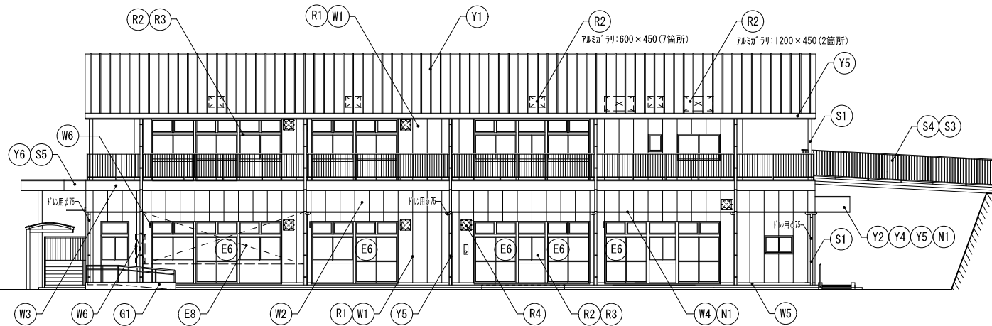
【改修後】西面 立面図 S=1:150
