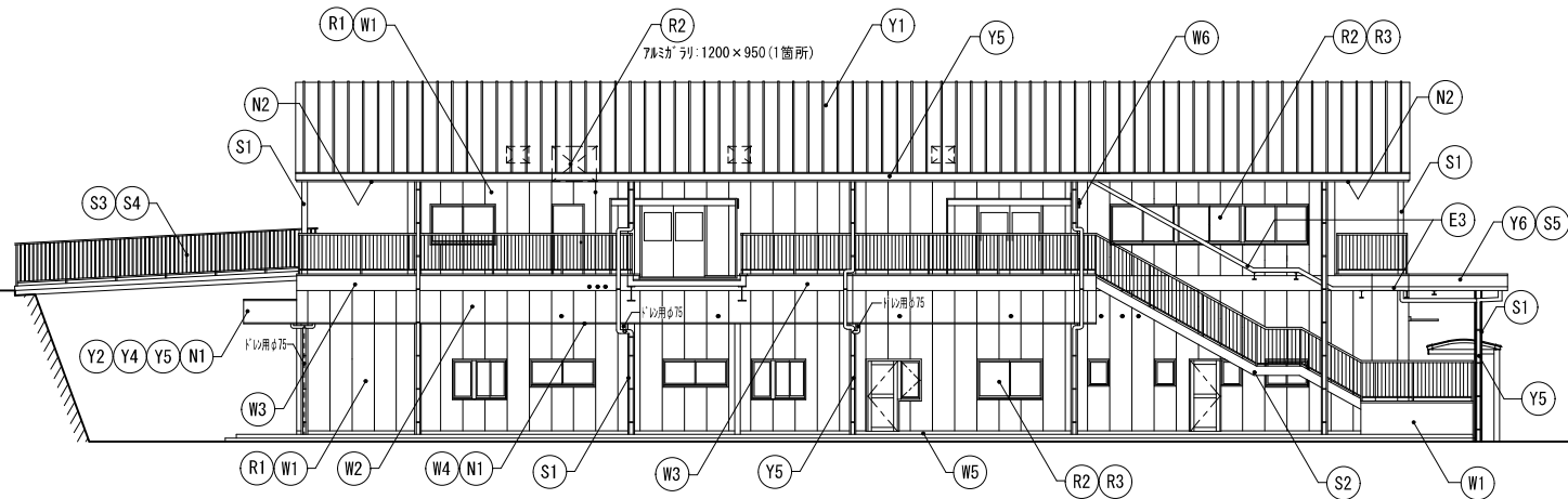
【改修後】東面 立面図 S=1:150
