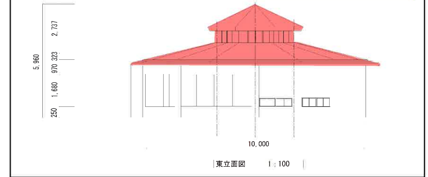
浴室棟 立面図
