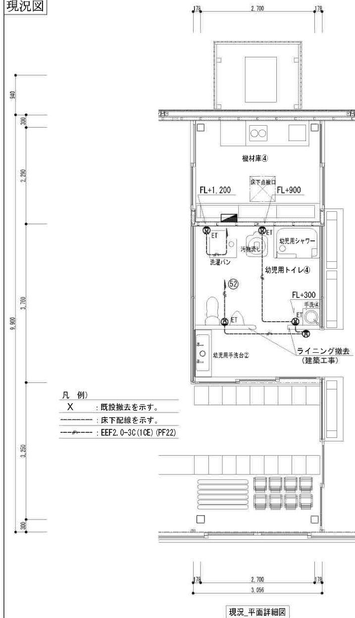
現況_平面詳細図
