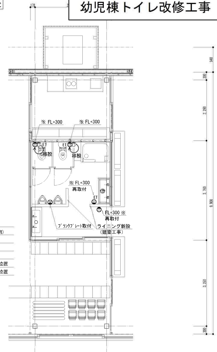
計画_平面詳細図
