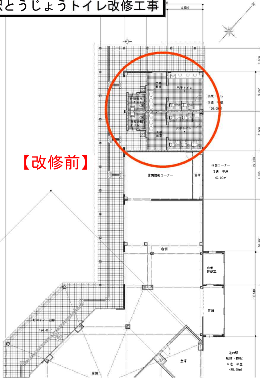
平面図（改修前） 1/100
