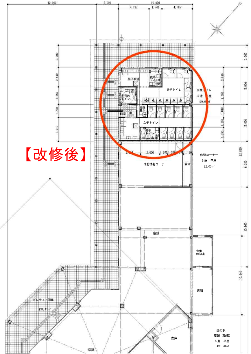
平面図（改修後） 1/100
