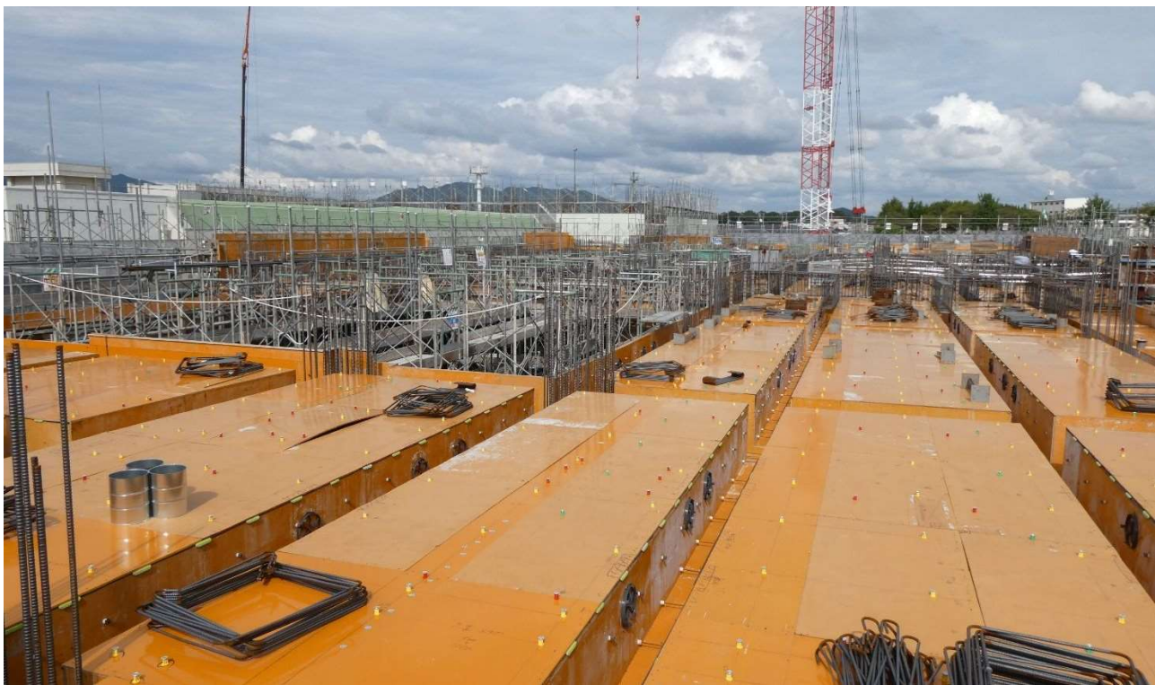
②増築校舎棟 3階 床型枠建込状況（令和5年8月18日撮影）
