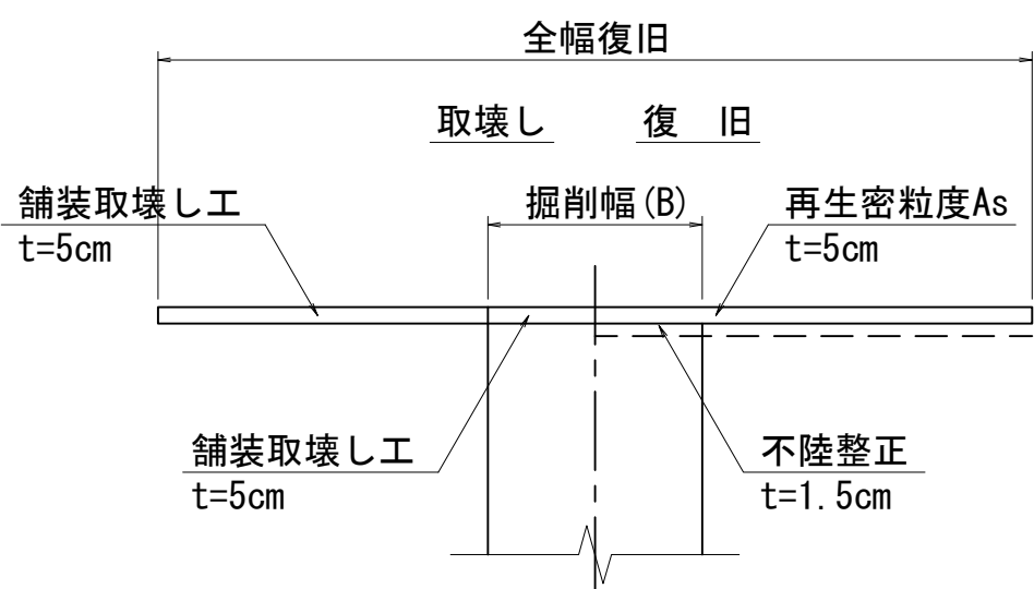
舗装構成図
