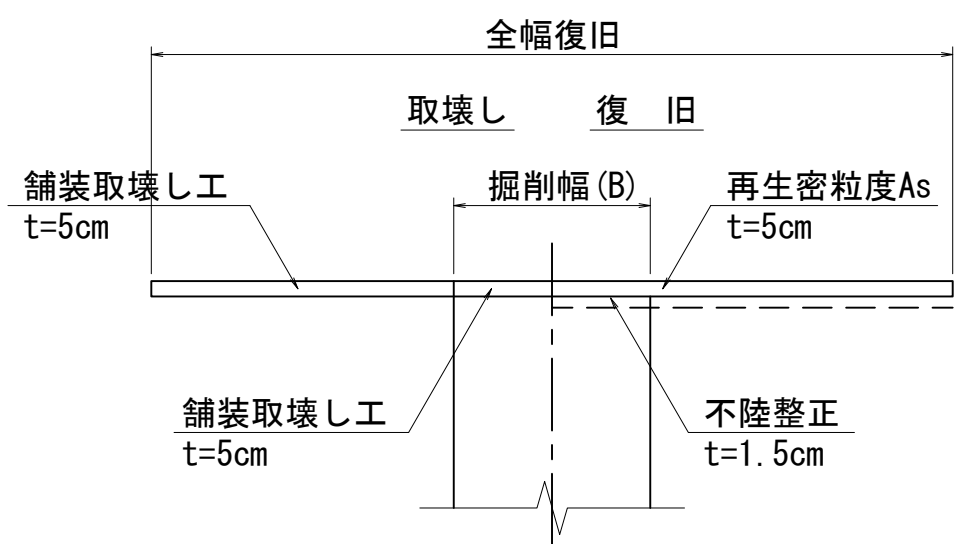
舗装構成図
