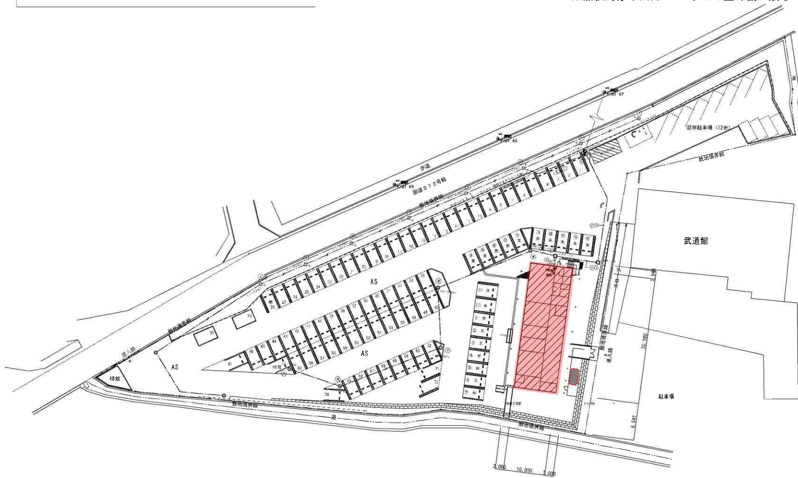
改修後 配置図 S=1,300
