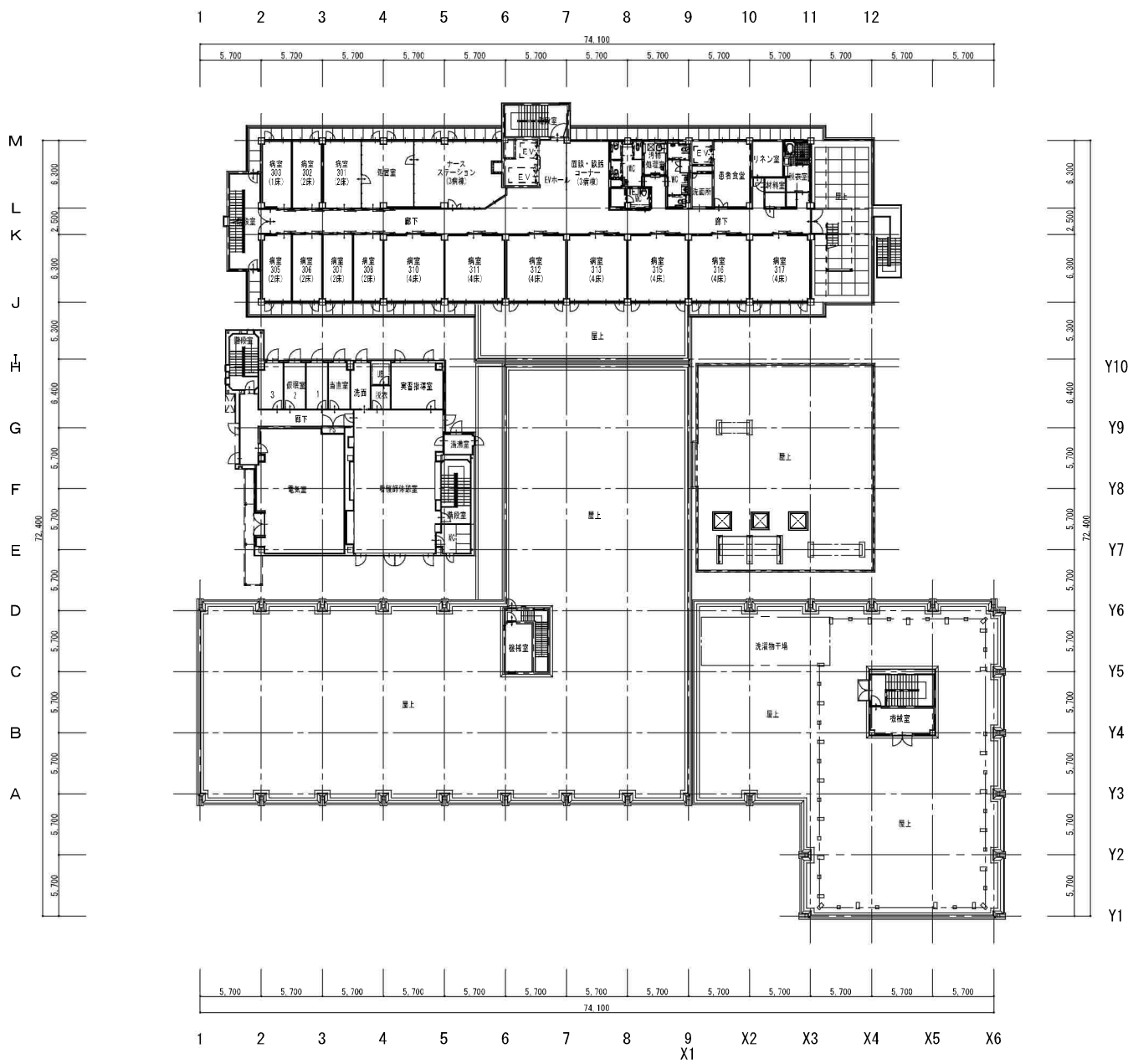
3階平面図 (S=1/400)
