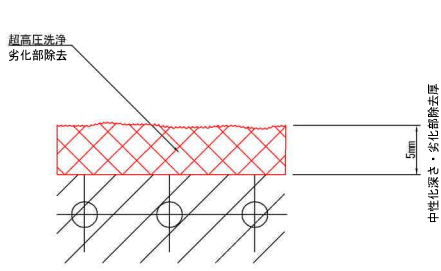
補修前 断面図
