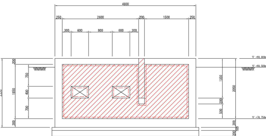
A-A 断面図
