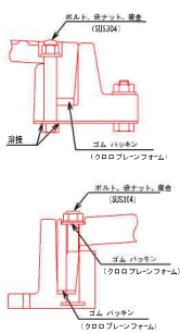
参考図-2 蓋ロック機構断面図
