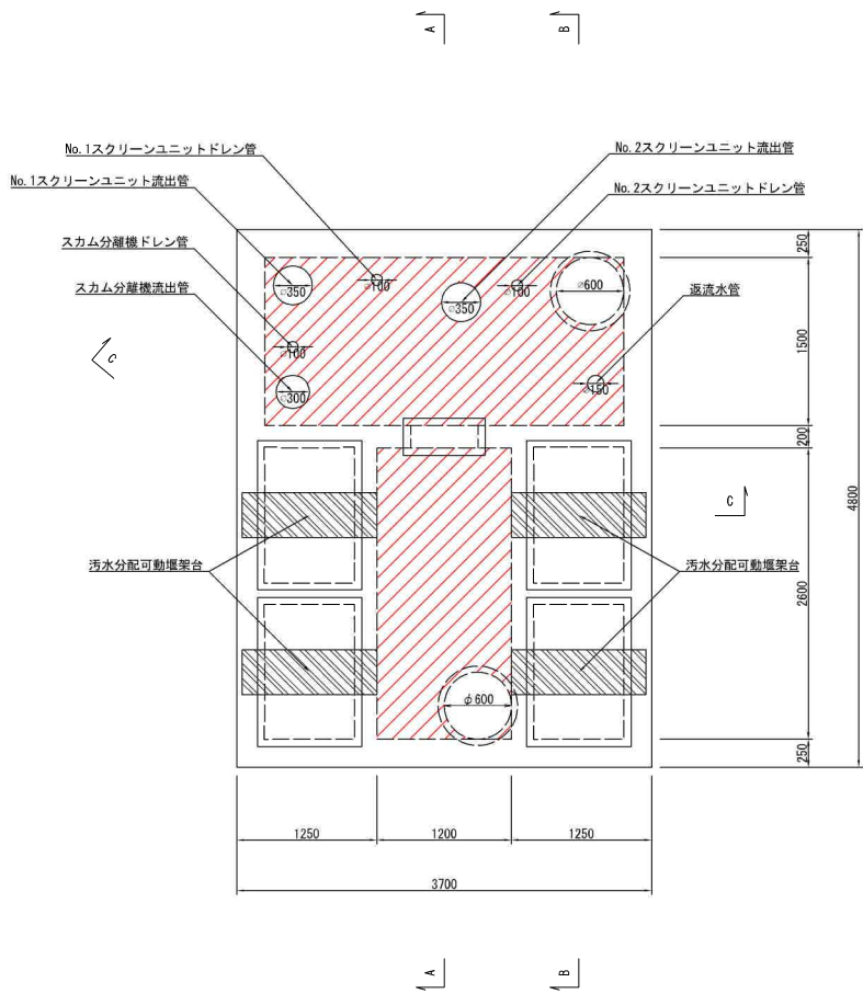
上部平面図
