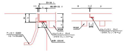
蓋形式: タイプII
