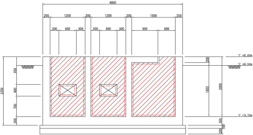
B-B 断面図
