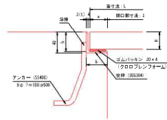
蓋形式: タイプI
