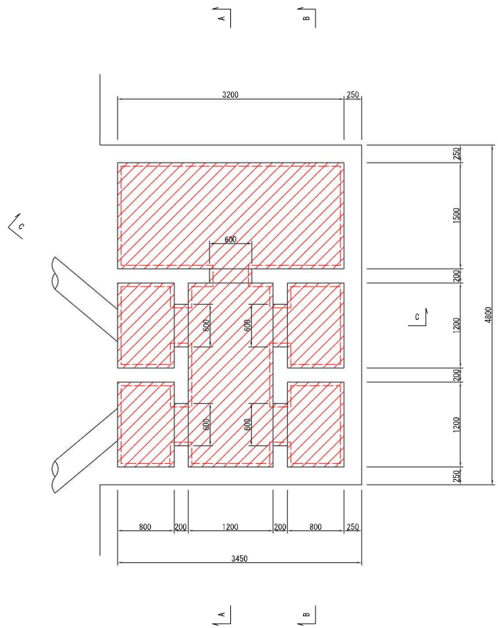
水路部平面図
