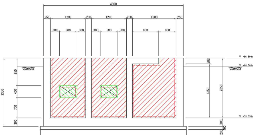
B-B 断面図
