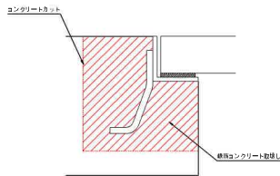
既設受枠除去標準図
