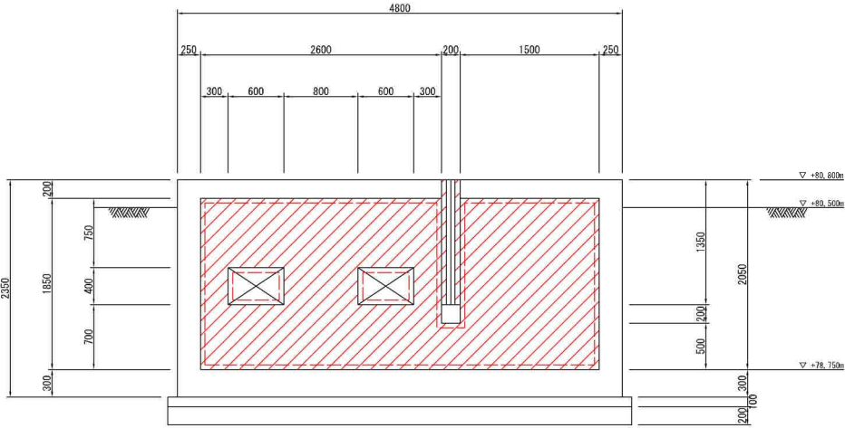
A-A 断面図
