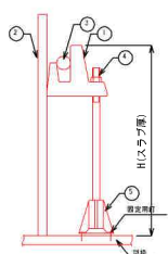
参考図-1 受枠施工断面図
