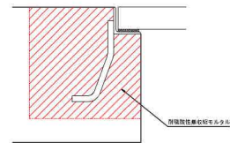
受枠更新標準図
