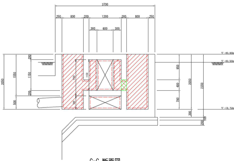
C-C 断面図
