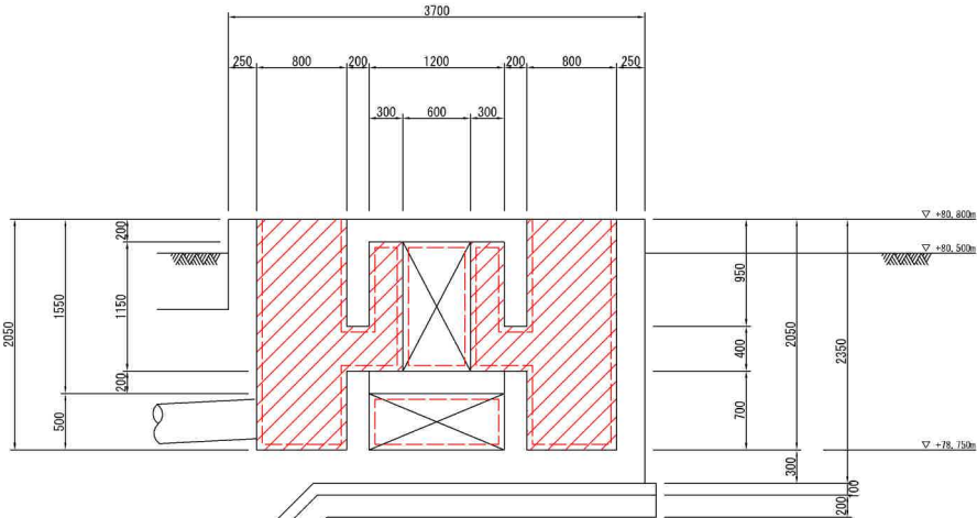
A-A 断面図
